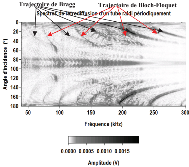
Figure 13: Plan spectral des signaux diffusés par un tube d'acier inoxydable comportant 49 raidisseurs transversaux.
