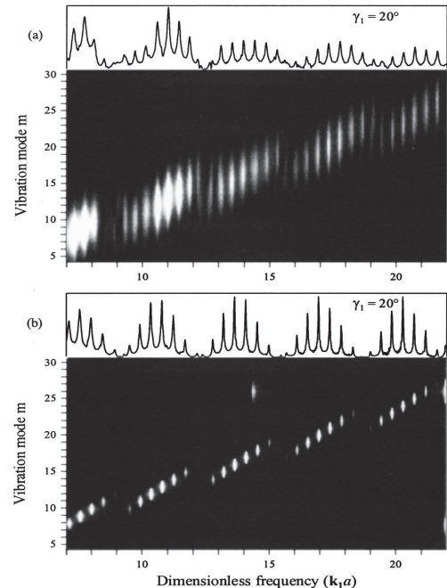
Figure 9: Identification du mode m sur la longueur du tube limité pour un angle d'incidence de 20^\circ . (a) résultats expérimentaux et (b) résultats théoriques.
