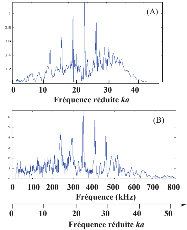
Figure 15: (A) : spectre de résonance de la cible en plein eau ; (B) : spectre de la cible enfouie dans le sable gorgé d'eau.
