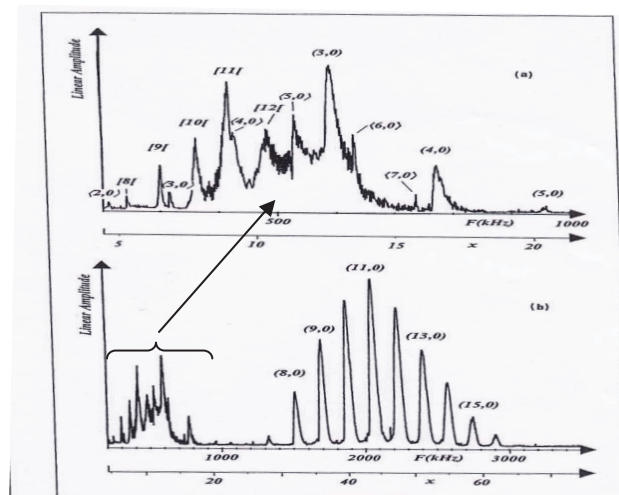
Figure 5: Spectre de résonance pour une incidence \alpha = 5^\circ ; (A) : Loupe en basse fréquence réduite ( 5 < ka < 20 ) ; (B) : signal total dans la bande 7-75.
