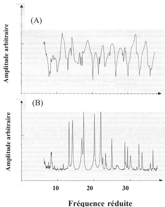
Figure 2: (A) spectre de rétrodiffusion, (B) spectre de résonance.
