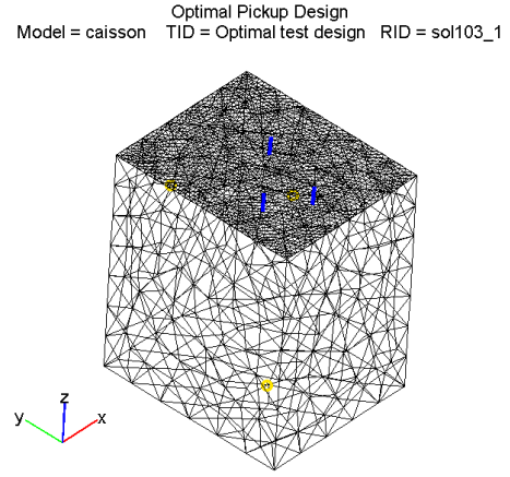
FIGURE 6 – Positionnement des capteurs
