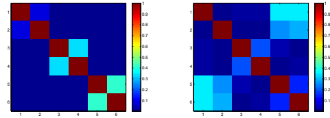
FIGURE 7 – Matrices d'AutoMAC sur les 6 premiers modes, lorsque tous les DDL sont observés, et lorsque les 6 DDL choisis sont observés
