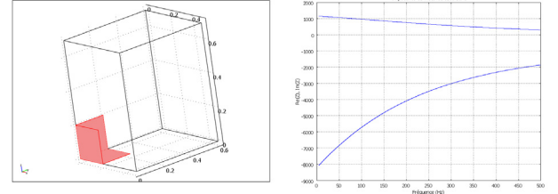
FIGURE 1 – a) Cavit   et emplacements du mat  riau, b) Imp  dance du mat  riau
