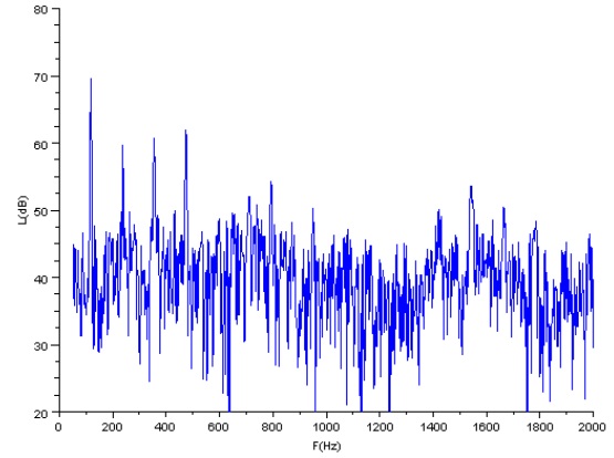
FIGURE 5 – Spectres en bandes fines du scooter Q circulant à 45 km/h.
