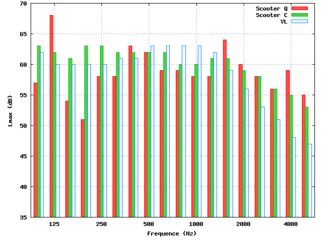
FIGURE 4 – Spectre en linéaire correspondant à une valeur de 70 dB(A) de deux scooters et un VL moyen.
