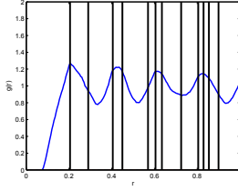
FIG. 7 – RDF pour une répartition périodique perturbée \phi = 5\%
