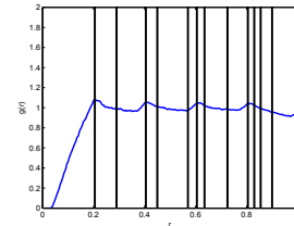
FIG. 6 – RDF pour une répartition périodique perturbée \phi = 1\%
