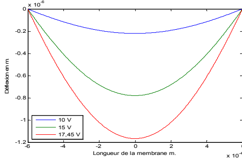
Figure 9 : Déflexion du centre de la membrane
