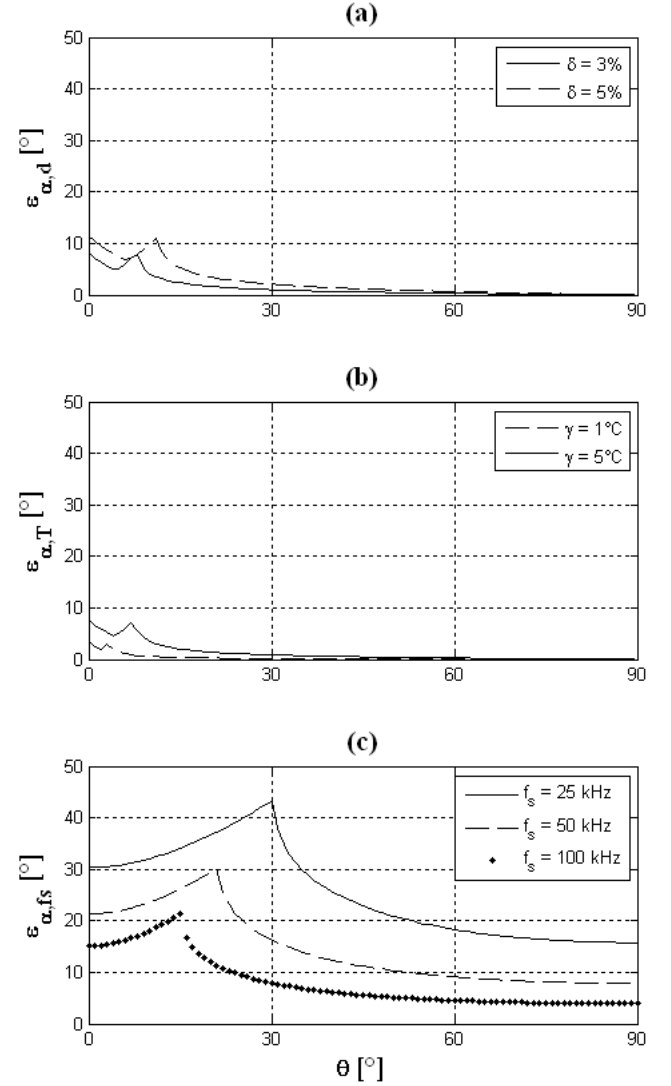
FIGURE 5 – Imprécision angulaire \epsilon_{\alpha} théorique pour une antenne de deux microphones séparés par une distance d = 20 cm en fonction (a) : de différentes fréquences d'échantillonnage, (b) : de différentes tolérances de distance, (c) : de différentes tolérances en température.
