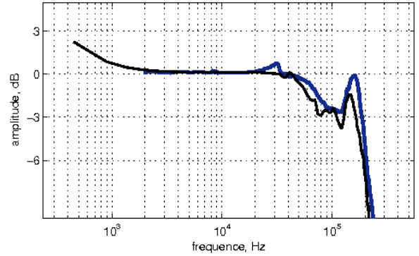
FIG. 7: Réponse fréquentielle d'un microphone Brüel & Kjær 1/8'' type 4138 estimée par la mesure microphonique de l'onde en N lorsque le micro est bafflé et sans grille (noir), comparée à la réponse fréquentielle issue de la calibration par le fabricant en utilisant la méthode de la grille électrostatique (bleu).
