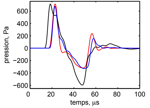
FIG. 6: Forme de l'onde mesurée par un microphone 1/8'' en incidence normale pour trois montages différents. En noir : monté sans grille de protection dans un baffle pour rejeter la diffraction; en bleu : sans baffle, sans grille; en rouge : sans baffle, avec grille de protection.
