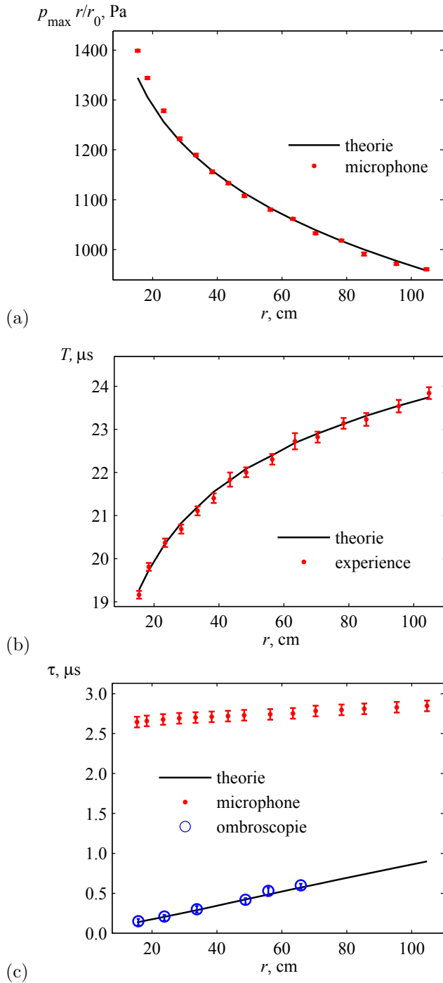
FIG. 3: Comparaison de mesures et de prédictions théoriques en fonction de la distance à la source.
