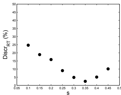
Figure 8 : Evolution de l'erreur \text{Disc}_{\text{RT}} en fonction de la diffusion pour la bande de tiers d'octave 2500 Hz.
