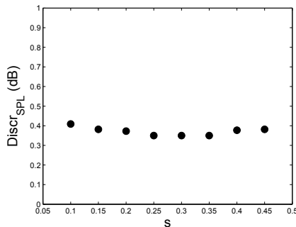
Figure 7 : Evolution de l'erreur \text{Disc}_{\text{SPL}} en fonction de la diffusion pour la bande de tiers d'octave 2500 Hz.
