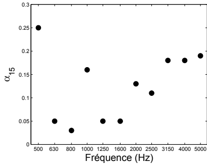
Figure 6 : Valeurs de l'absorption pour s=0,15 minimisant l'erreur \text{Disc}_{\text{SPL}} (par bande de tiers d'octave).
