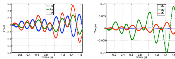
FIGURE 15 – Torseur des efforts globaux en O
