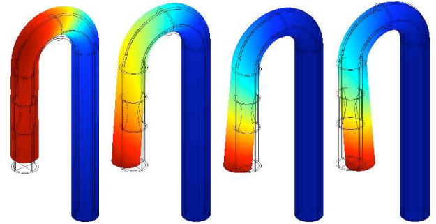
FIGURE 17 – Condition en pression. Déformées à t = 0.1, 0.2, 0.3, 0.8 (s) pour une conditions
