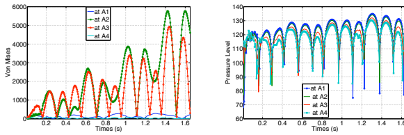
FIGURE 14 – Von Mises et niveau sonore aux points A_i
