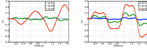
FIGURE 4 – Composantes u et w de \mathbf{u} aux points A_i .
