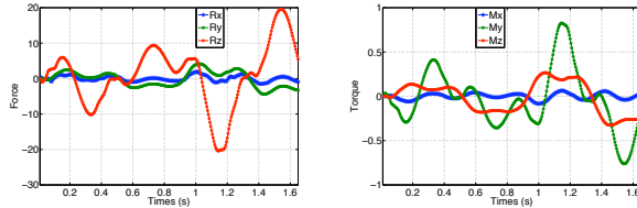
FIGURE 6 – Le torseur des efforts globaux en O
