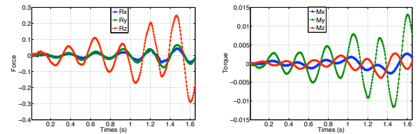
FIGURE 9 – Le torseur des efforts globaux en O
