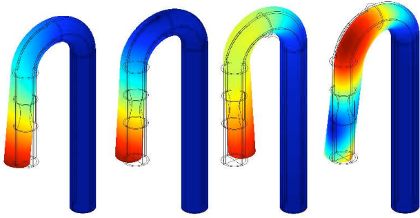
FIGURE 2 – Les 4 premières formes modales dans le cas sténosé
