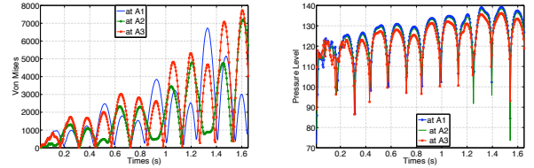
FIGURE 8 – Von Mises et niveau sonore aux points A_i
