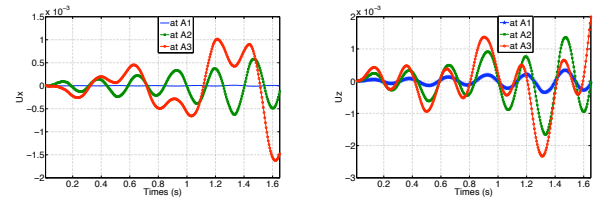
FIGURE 7 – Composantes u et w de \mathbf{u} aux points A_i .
