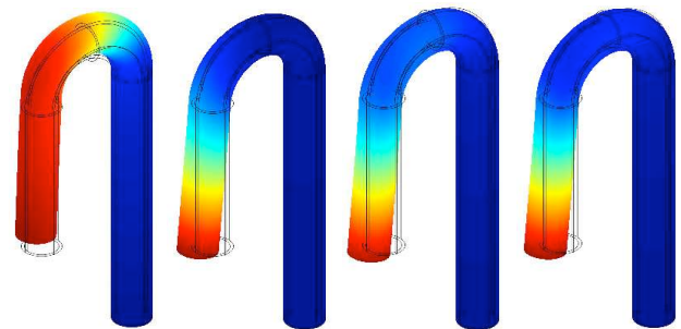
FIGURE 18 – Condition en accélération. Déformées à t = 0.1, 0.2, 0.3, 0.8 (s)
