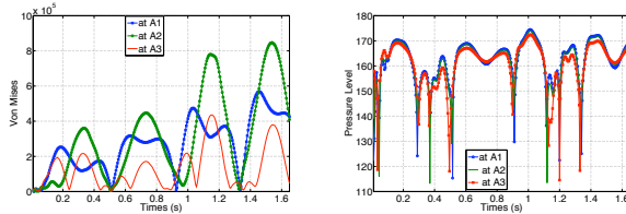
FIGURE 5 – Von Mises et niveau sonore aux points A_i
