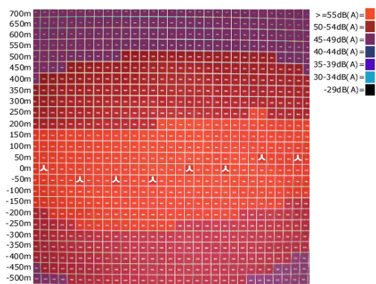
Figure 6. Niveaux de bruit de fonctionnement [Association des fabricants danois de turbines éoliennes]
