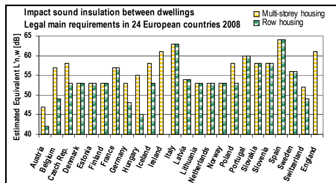
Figure 4 : Synthèse, pour 24 pays, des exigences minimales, exprimé en L'_{n,w} équivalent (valeur parfois estimée), pour l'isolation au bruit de choc entre appartements, respectivement entre maisons mitoyennes. Tirée de [2].
