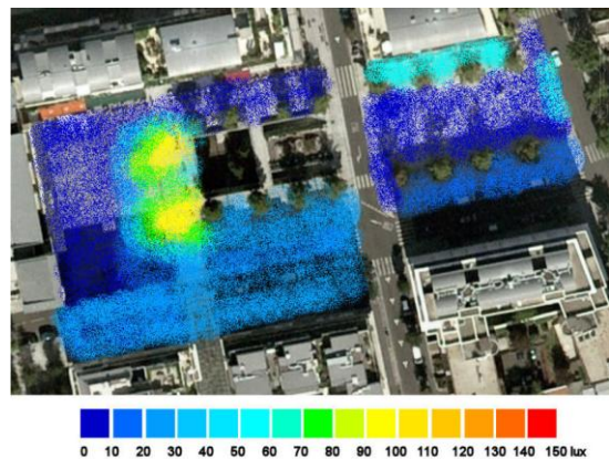
Figure 2 : cartographie des éclairagements horizontaux mesurés à 1m de hauteur Grand Place, Boulogne Billancourt
