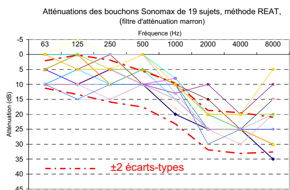
Figure 6 : Comparaison des atténuations du bouchon Sonomax de chaque participant avec la spécification \pm 2 écarts-types du fabricant.
