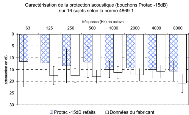
Figure 4 : Comparaison des atténuations moyennes et écarts-types des bouchons Protac (-15dB) refaits
