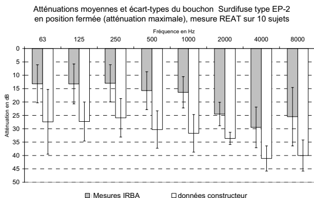
Figure 5 : Comparaison des atténuations du bouchon personnalisé en acrylique
