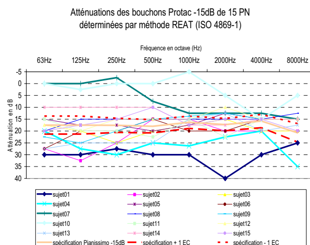
Figure 3 : Atténuations des bouchons personnalisés en silicone de chaque PN, mesurées à l'IRBA
