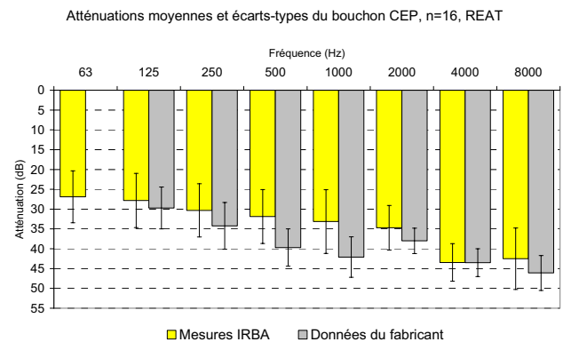
Figure 7 : Comparaison des atténuations moyennes et des écarts-types des bouchons CEP
